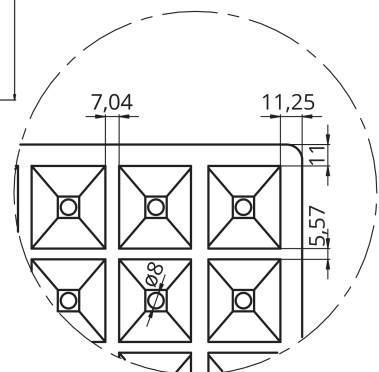
DETALLE A
