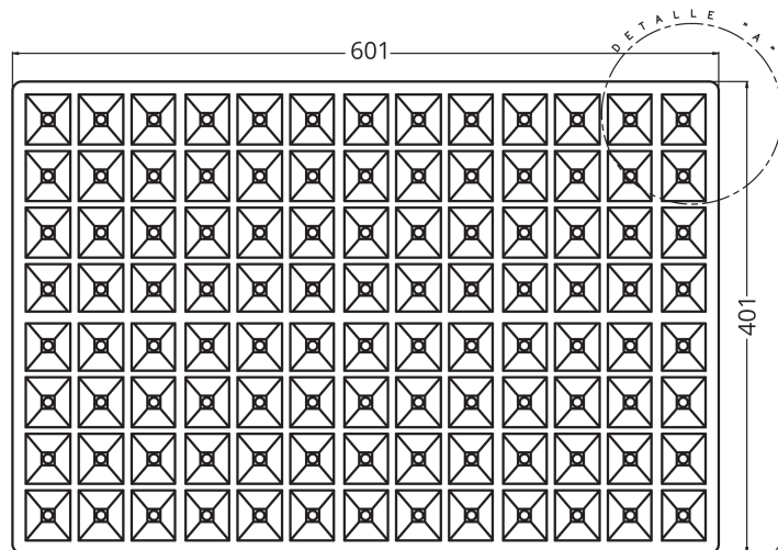
PLANTA SUPERIOR
