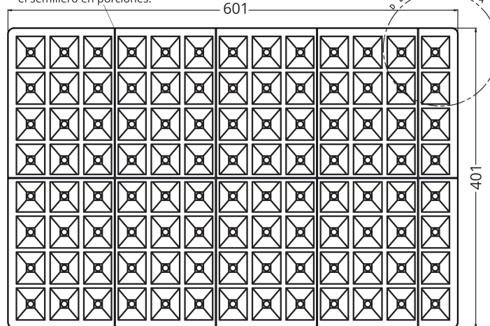
PLANTA SUPERIOR
