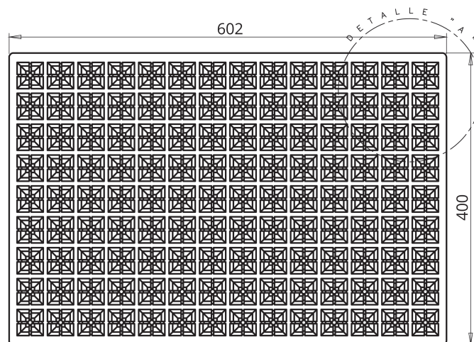
PLANTA SUPERIOR
