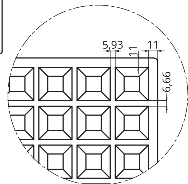
DETALLE A
