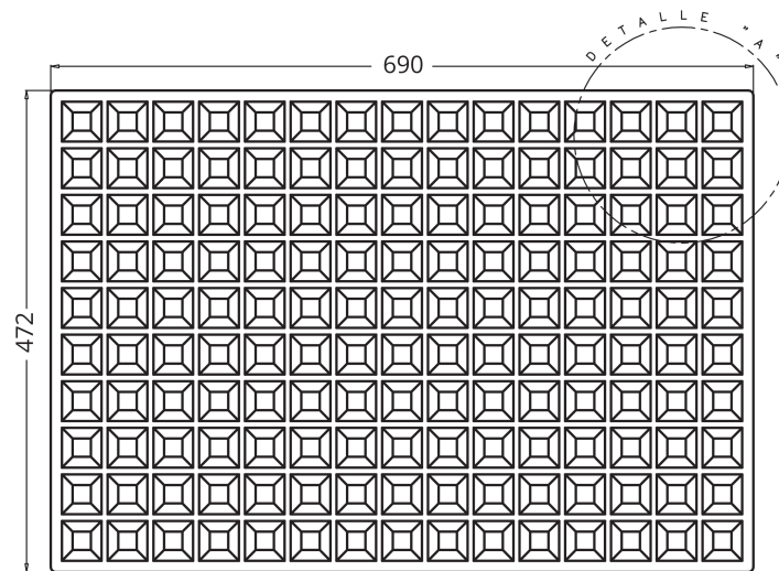
PLANTA SUPERIOR
