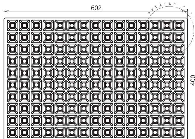
PLANTA SUPERIOR
