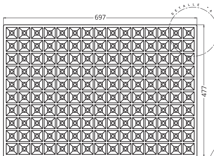
PLANTA SUPERIOR
