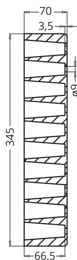
SECCIÓN A-A
