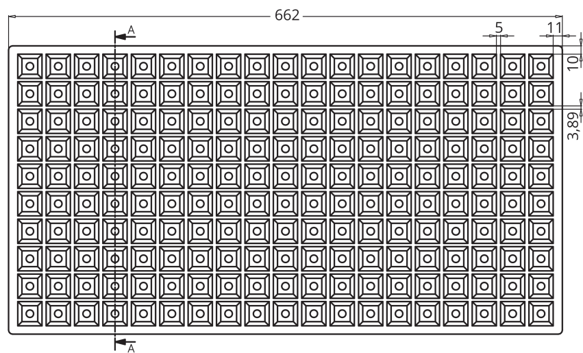
PLANTA SUPERIOR
