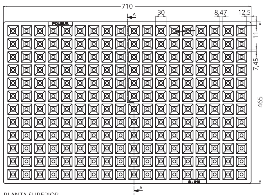
PLANTA SUPERIOR
