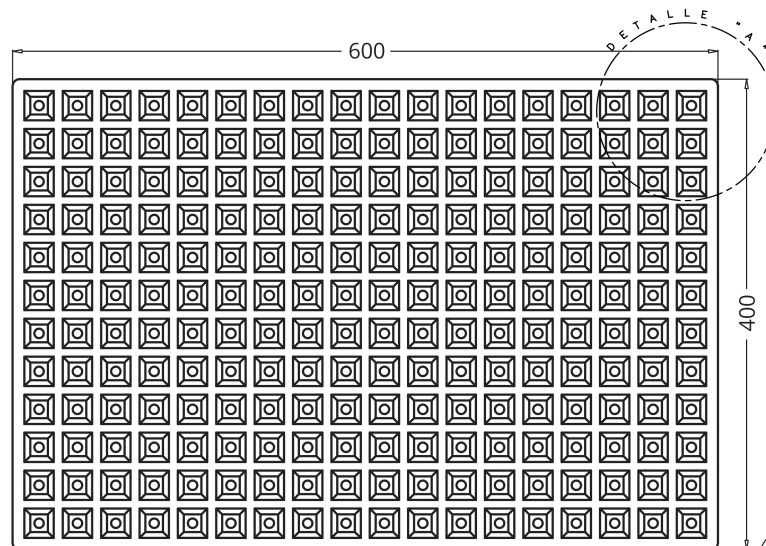
PLANTA SUPERIOR
