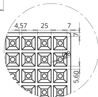
DETALLE A
