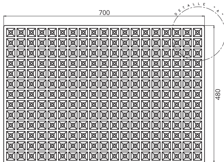
PLANTA SUPERIOR
