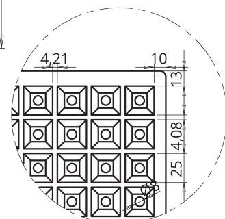
DETALLE A
