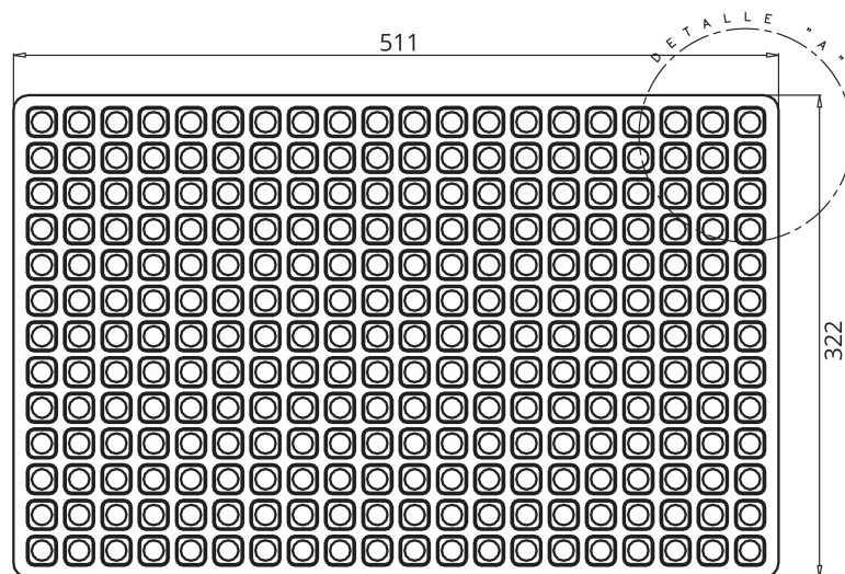
PLANTA SUPERIOR
