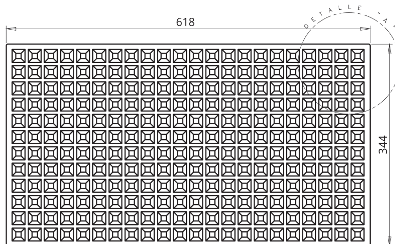
PLANTA SUPERIOR
