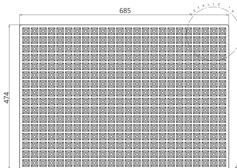
PLANTA SUPERIOR
