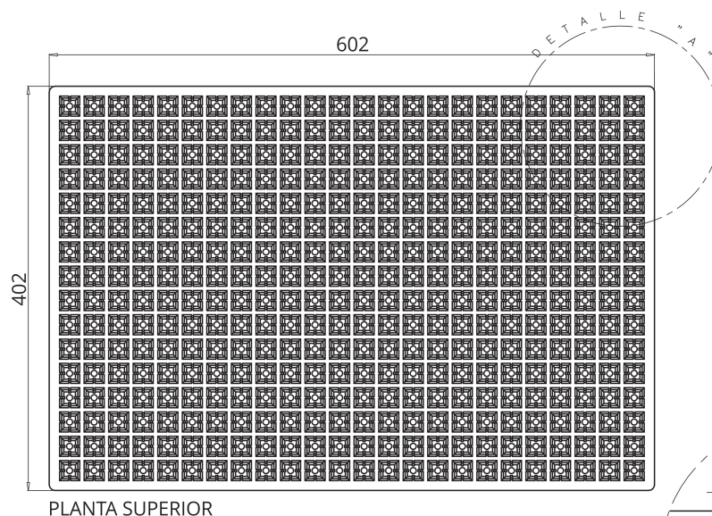
PLANTA SUPERIOR
