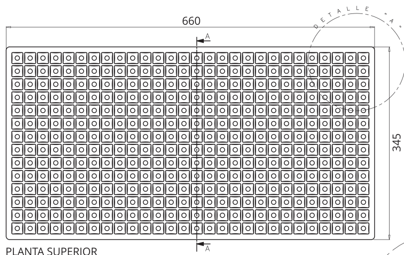
PLANTA SUPERIOR
