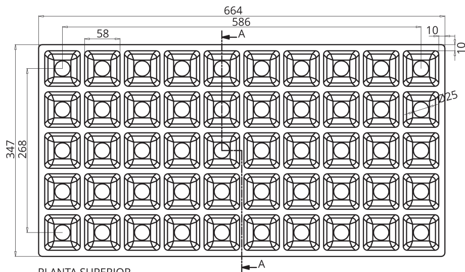
PLANTA SUPERIOR
