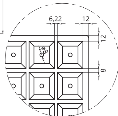
DETALLE A
