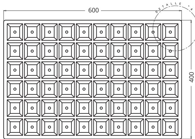
PLANTA SUPERIOR
