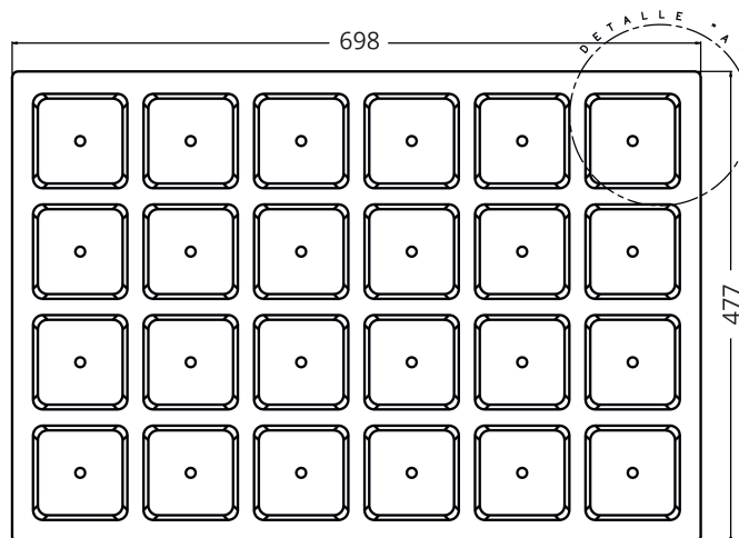
PLANTA SUPERIOR
