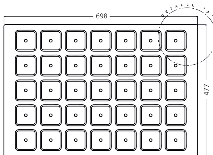
PLANTA SUPERIOR
