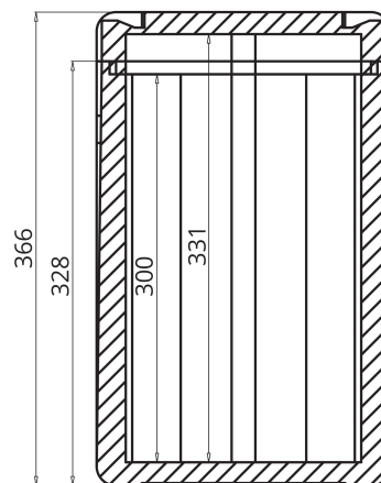
Sección del Conjunto
