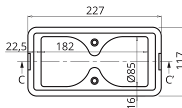
Planta Superior (Envase)
