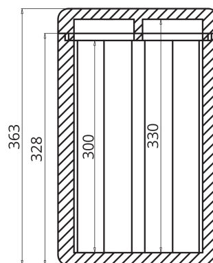
Sección del conjunto
