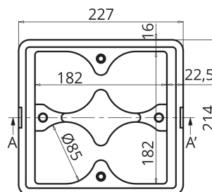
Planta Superior (Envase)
