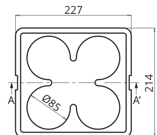
Planta Inferior (Tapa)
