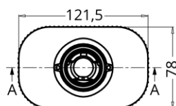
PLANTA SUPERIOR
