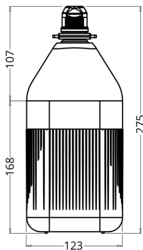
ALZADO FRONTAL
