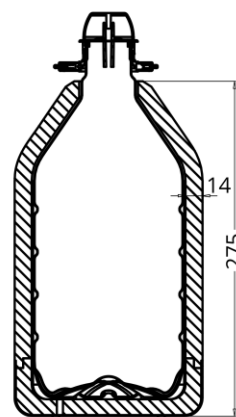
SECCION A-A
