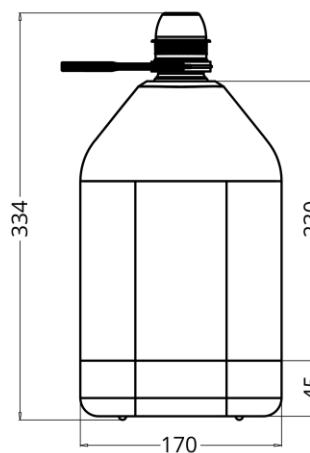
ALZADO FRONTAL
