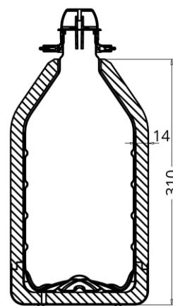
SECCION A-A
