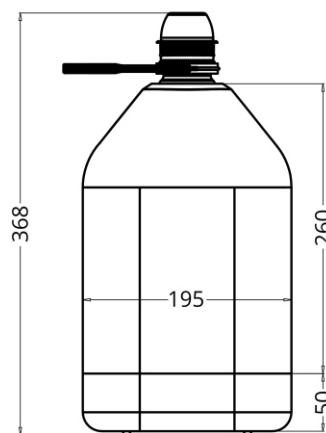
ALZADO FRONTAL
