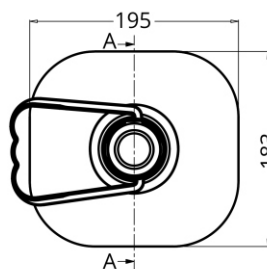
PLANTA SUPERIOR
