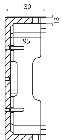
SECCION B-B
