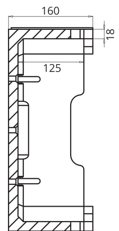
SECCION B-B
