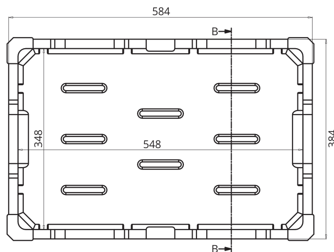
PLANTA SUPERIOR
