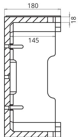
SECCION B-B
