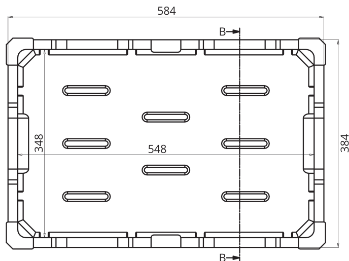
PLANTA SUPERIOR
