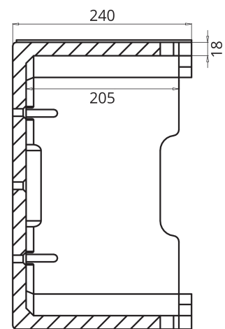
SECCION B-B
