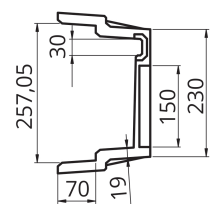
ALZADO LATERAL
