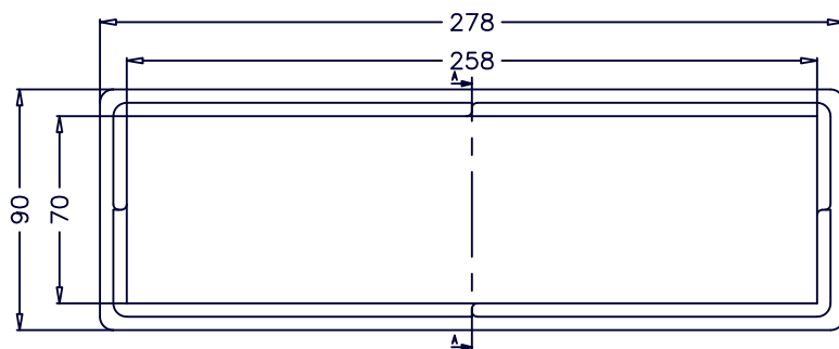
PLANTA SUPERIOR.
