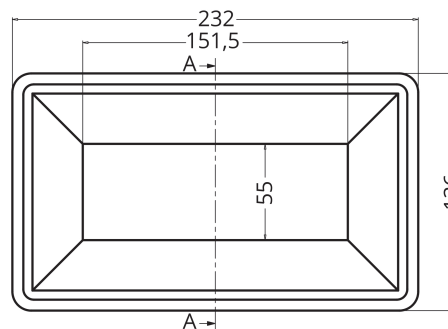
Planta Superior
