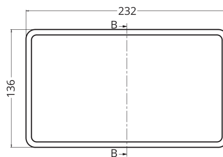
Planta Superior
