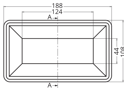
Planta Superior
