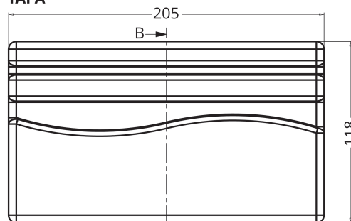
Planta Superior
