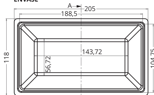
Planta Superior
