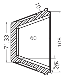
Sección A-A
