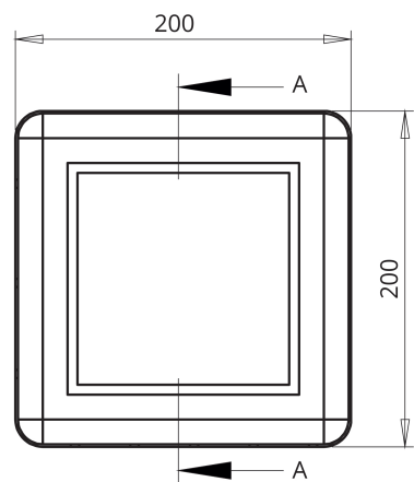
PLANTA SUPERIOR
