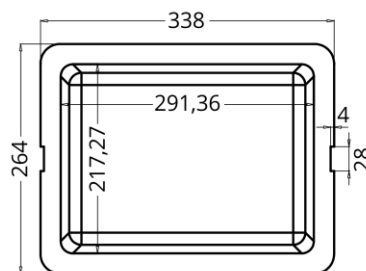
Planta Superior
