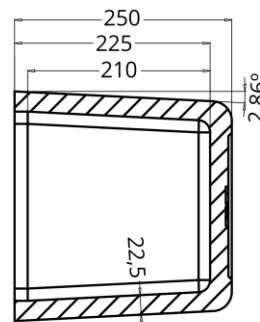
Sección A-A
