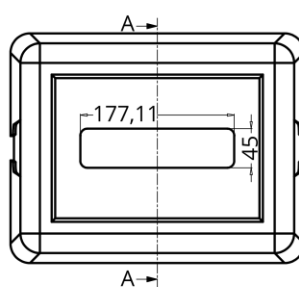
Planta Inferior
