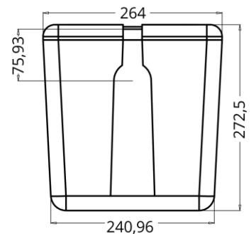
Alzado Lateral del Conjunto
