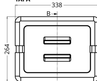
Planta Superior
