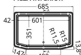
Planta Superior
