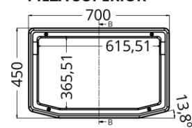
Planta Superior
