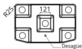
Planta Inferior
