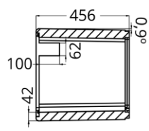
Sección B-B
