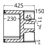
Sección A-A
