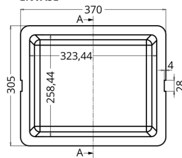
Planta Superior
