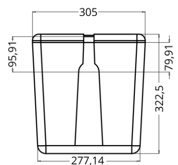
Alzado Lateral del Conjunto
