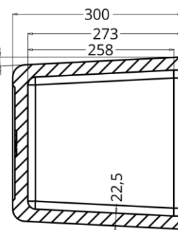
Sección A-A
