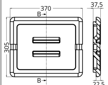
PLANTA SUPERIOR
