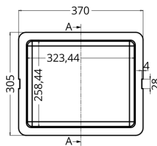
PLANTA SUPERIOR
