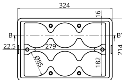
Planta Superior (Envase)
