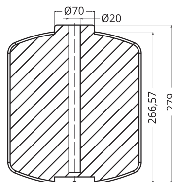
SECCION A-A
