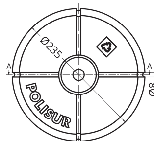
PLANTA SUPERIOR
