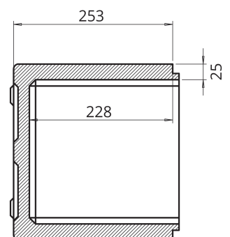
SECCION A-A
