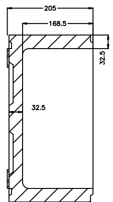
SECCIÓN A-A.
