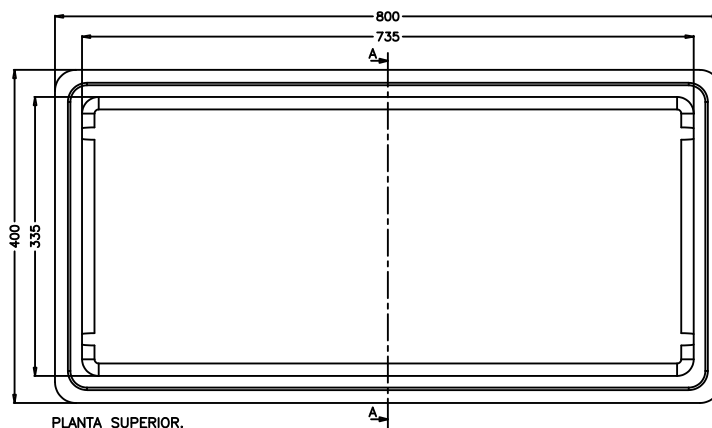
PLANTA SUPERIOR.
