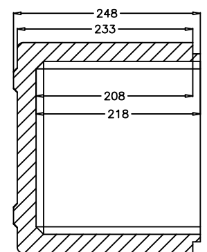
SECCIÓN A-A'.
