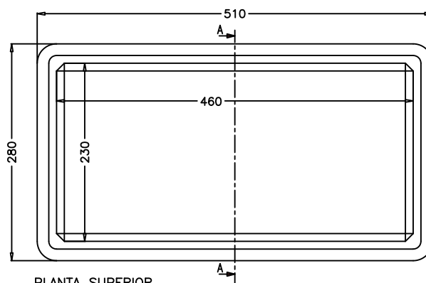
PLANTA SUPERIOR.
