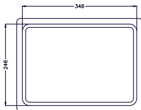
PLANTA INFERIOR.
