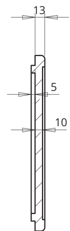
SECCION A-A Rv. Mayo 2020
