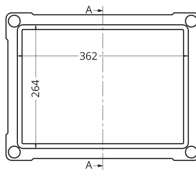
PLANTA SUPERIOR
