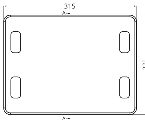
PLANTA SUPERIOR
