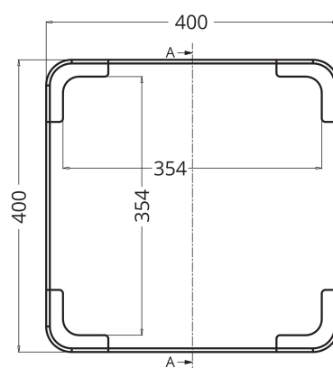
PLANTA SUPERIOR
